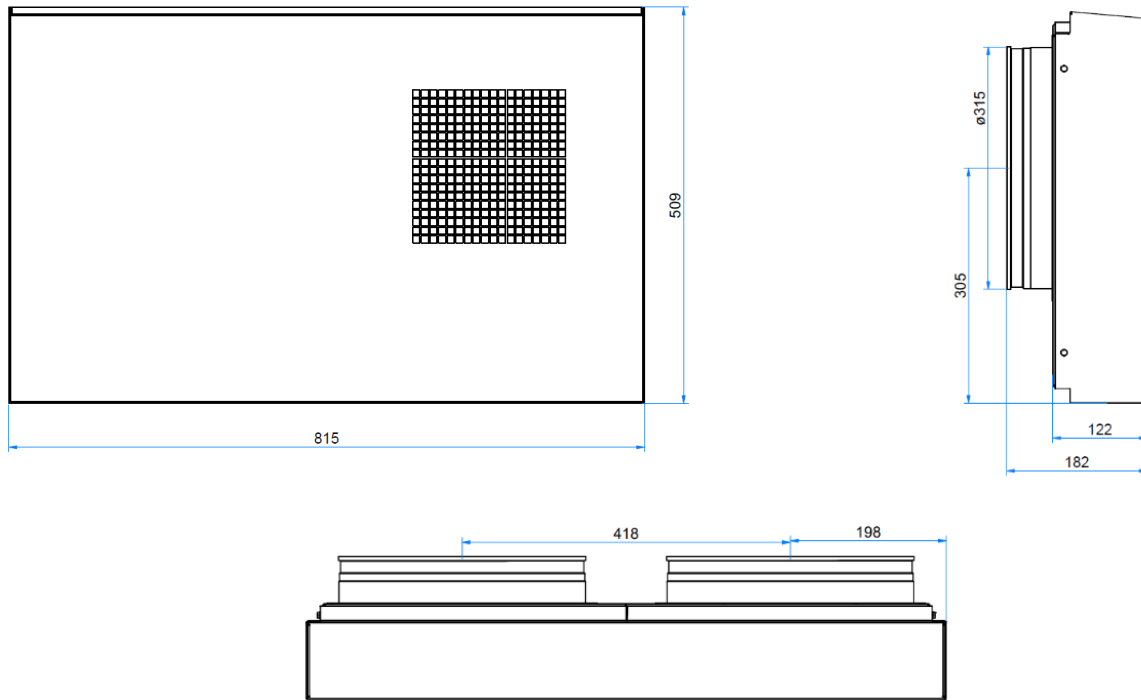
Figuur 2: Dimensionale tekening Muurafdekking
